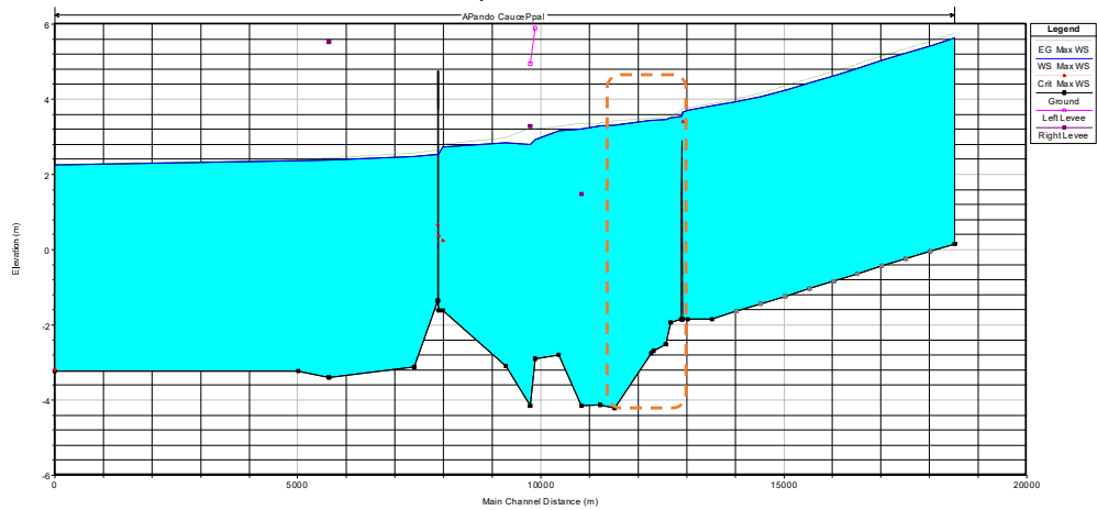
Figura 6.17 Perfil de flujo para una crecien de 10 años de periodo de retorno y nivel en el Río de la Plata de 10 años En línea punteada se observa la zona correspondiente al terreno
