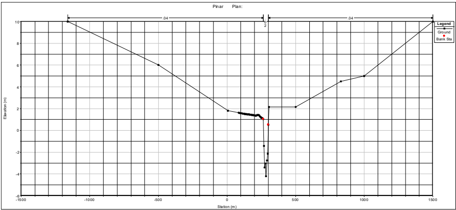
Figura 9.6 Sección 12
