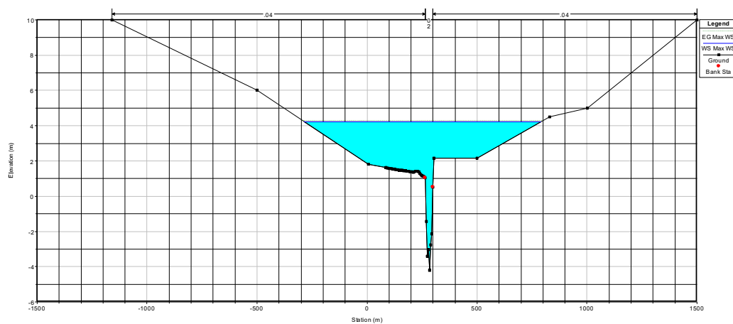
Figura 6.40 Sección inferior al predio. Cota máxima 4.28
