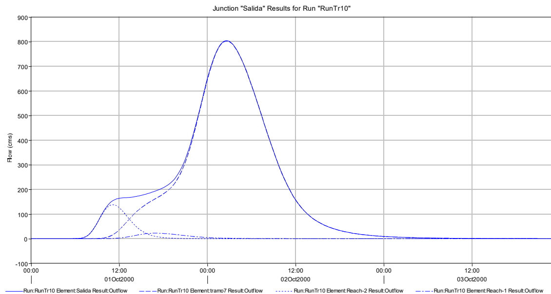
Figura 4.3 Hidrograma de cuenca de cabecera para Tr 10 años
