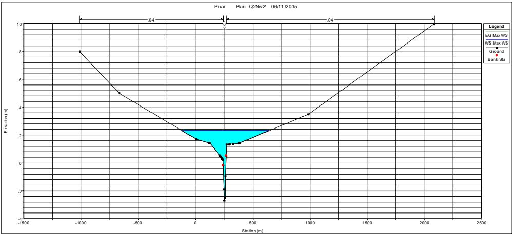
Figura 6.3 Sección inferior al predio. Cota máxima 2.43
