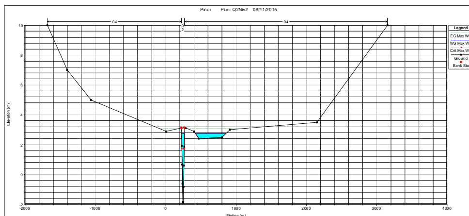
Figura 6.2 Sección superior al predio. Cota máxima 2.78 m
