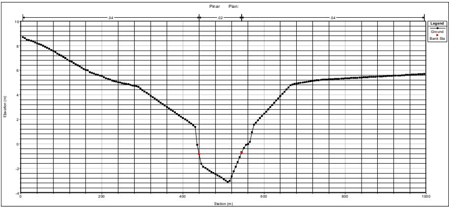
Figura 9.14 Sección 4
