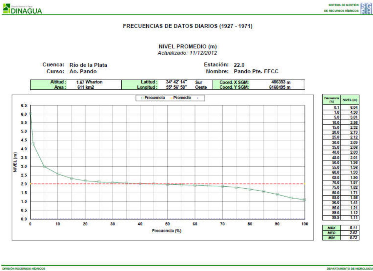
Figura 9.18 Curva de frecuencia de niveles diarios en la Estación Hidrométrica 22 (Pando Puente FFCC)
