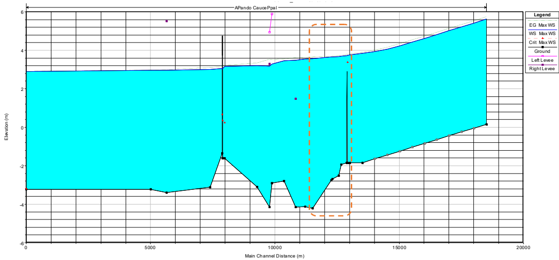
Figura 6.25 Perfil de flujo para una creciente de 10 años de período de retorno y nivel en el Río de la Plata de 100 años. En línea punteada se observa la zona correspondiente al terreno
