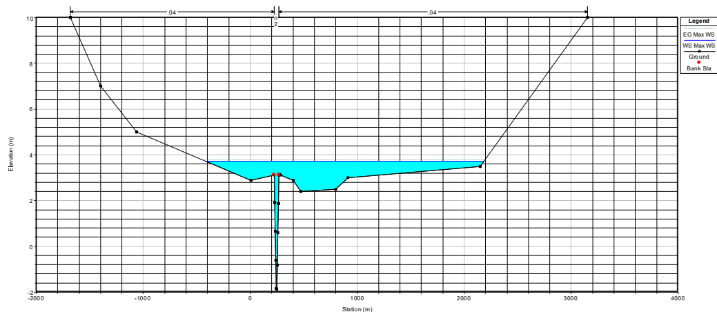
Figura 6.26 Sección superior al predio. Cota máxima 3.93 m
