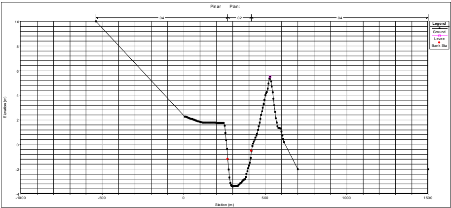
Figura 9.15 Sección 3
