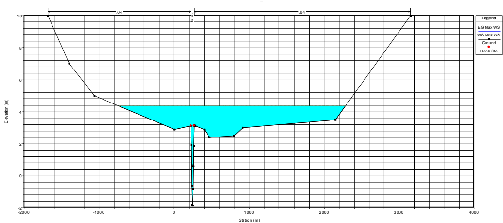
Figura 6.38 Sección superior al predio. Cota máxima 4.59
