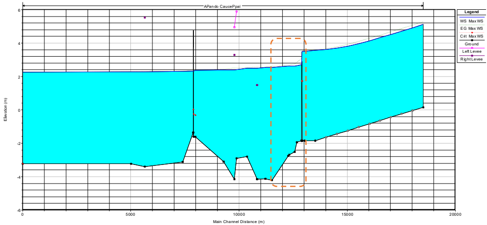
Figura 6.5 Perfil de flujo para una creciente de 2 años de período de retorno y nivel en el Río de la Plata de 10 años. En línea punteada se observa la zona correspondiente al terreno
