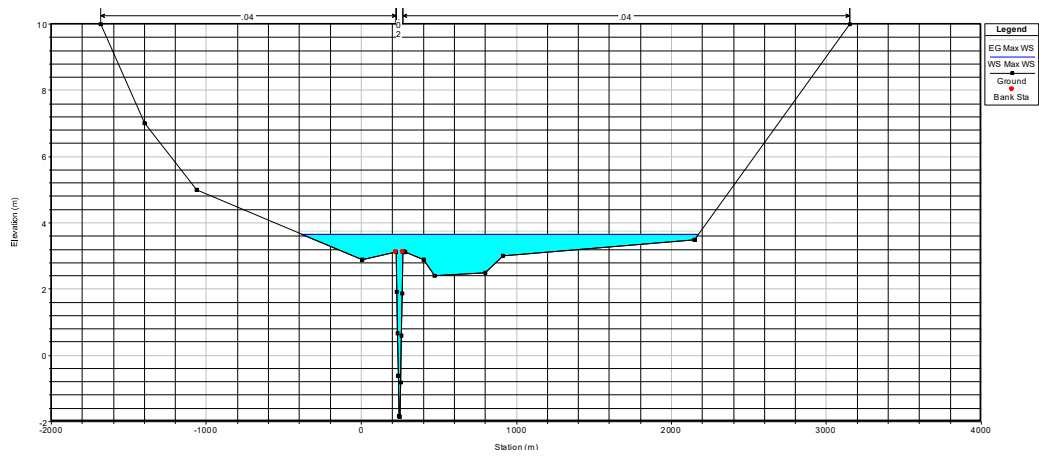
Figura 6.22 Sección superior al predio. Cota máxima 3.88
