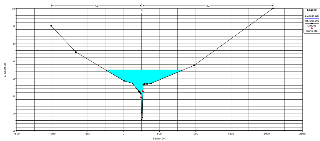
Figura 6.11 Sección central al predio. Cota máxima 2.96 m
