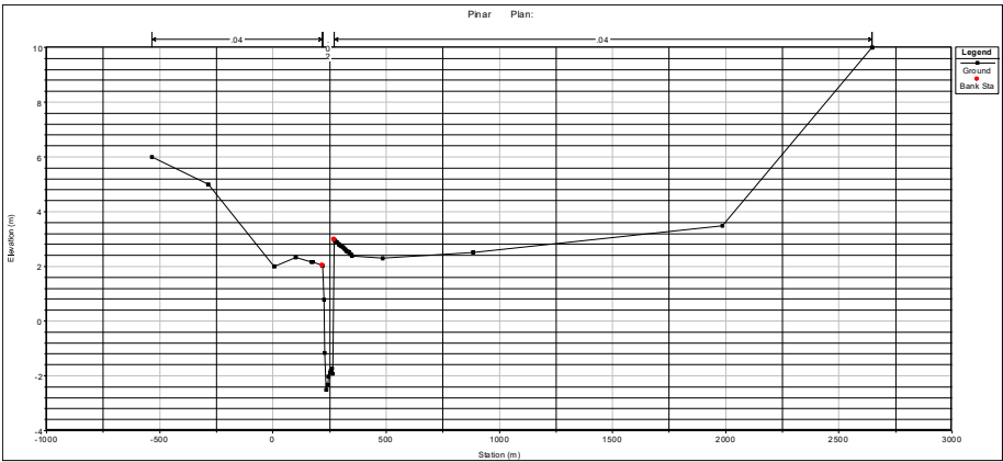
Figura 9.3 Sección 15
