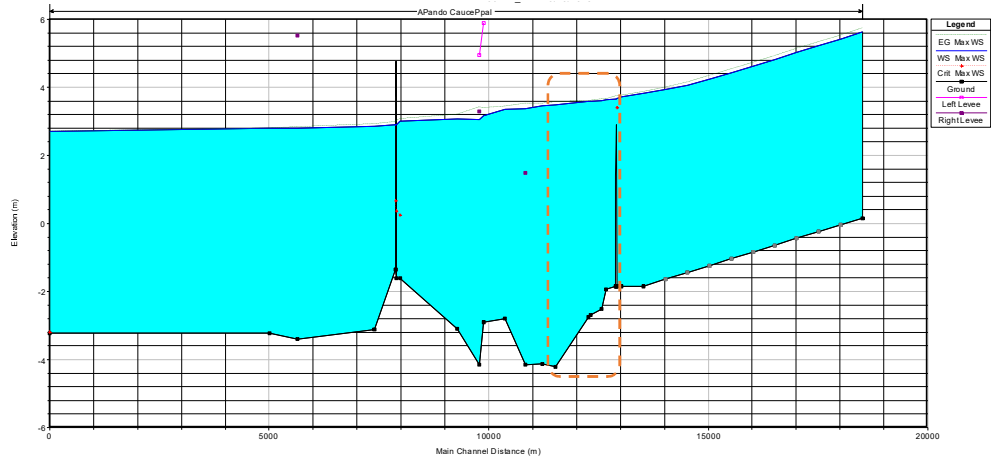
Figura 6.21 Perfil de flujo para una crecida de 10 años de período de retorno y nivel en el Río de la Plata de 50 años. En línea punteada se observa la zona correspondiente al terreno
