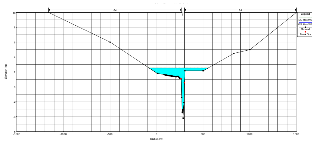
Figura 6.8 Sección inferior al predio. Cota máxima 2.58
