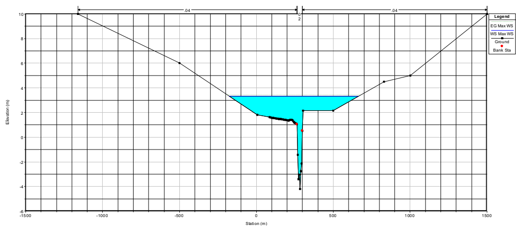
Figura 6.20 Sección inferior al predio. Cota máxima 3.35
