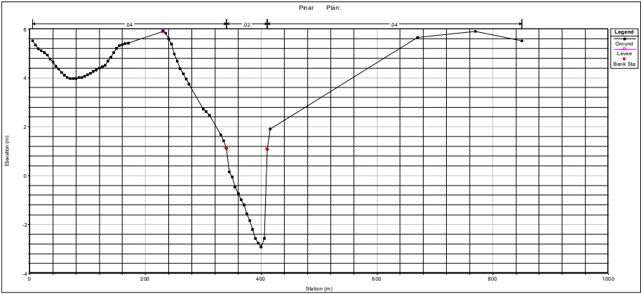
Figura 9.10 Sección 8
