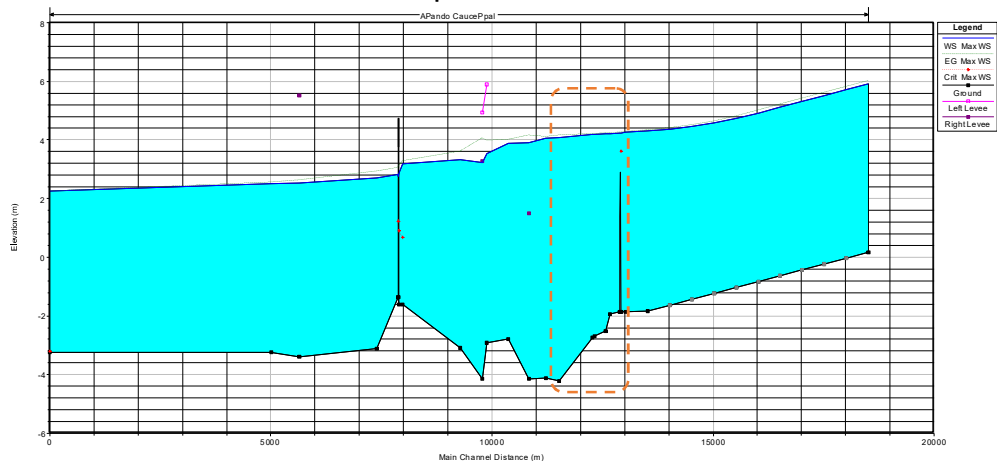
Figura 6.29 Perfil de flujo para una creciente de 100 años de periodo de retorno y nivel en el Río de la Plata de 10 años En línea punteada se observa la zona correspondiente al terreno
