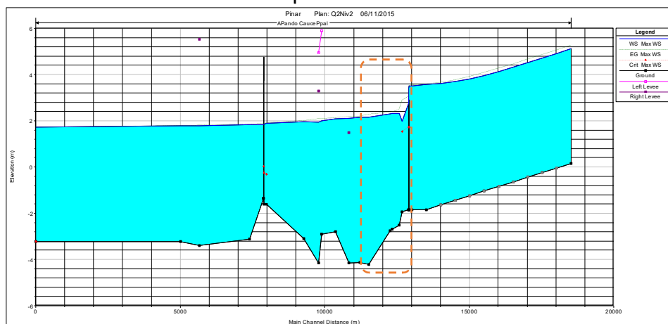
Figura 6.1 Perfil de flujo para una creciente de 2 años de período de retorno y nivel en el Río de la Plata de 2 años. En línea punteada se observa la zona correspondiente al terreno
