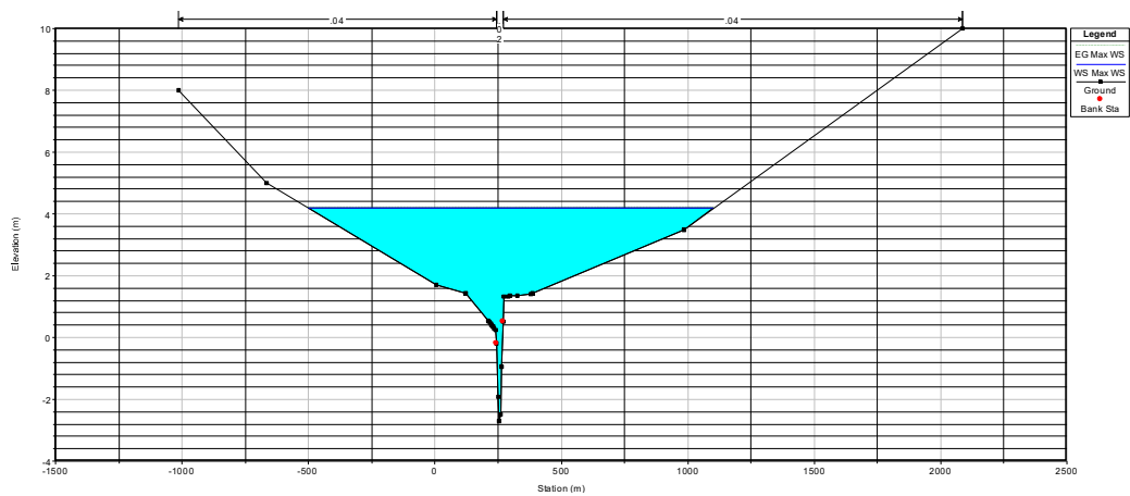
Figura 6.31 Sección central al predio. Cota máxima 4.38 m
