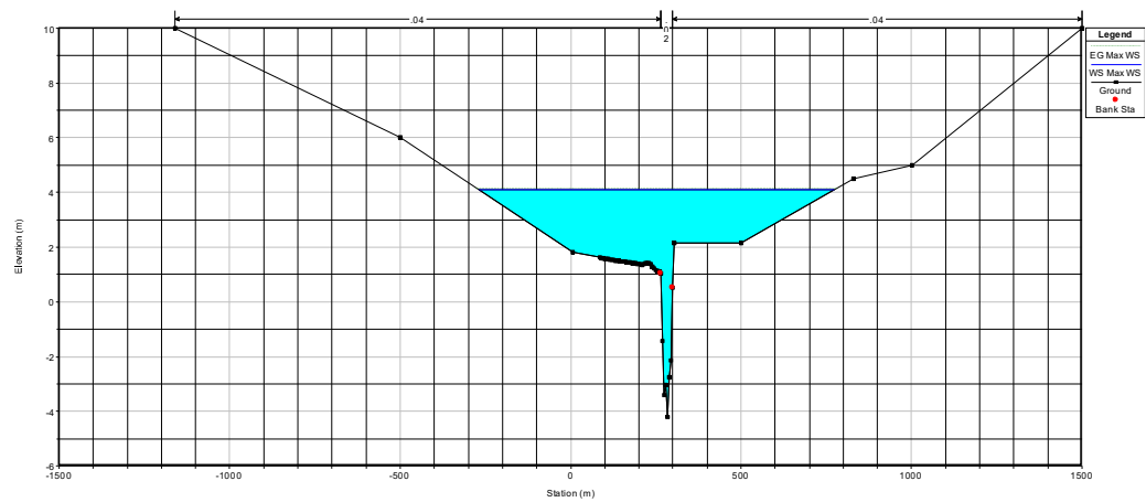
Figura 6.32 Sección inferior al predio. Cota máxima 4.14
