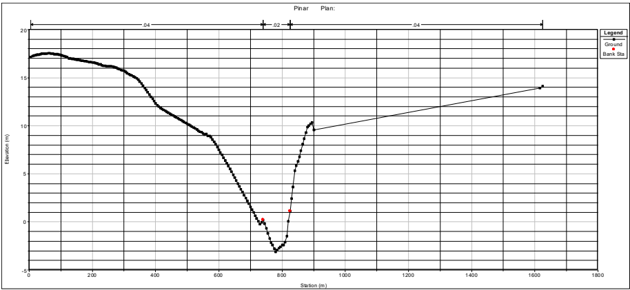
Figura 9.12 Sección 6
